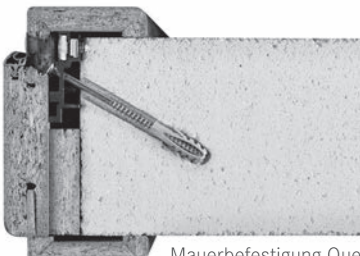
Mauerbefestigung Querschnitt
