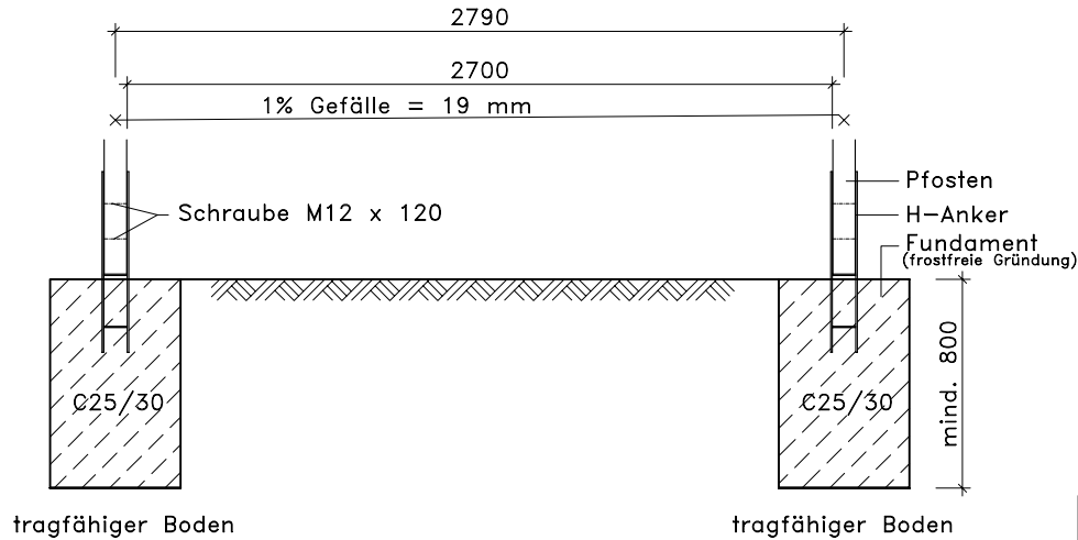
Schnitt B-B
