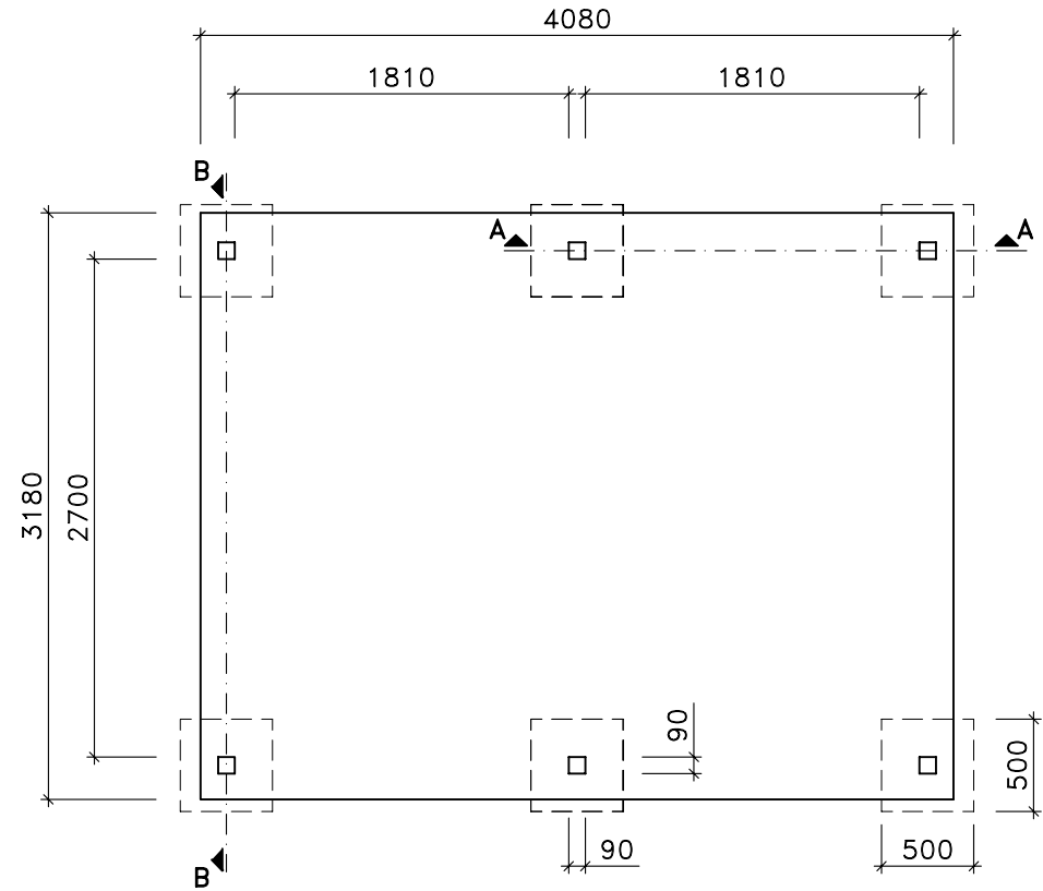
Grundriß
