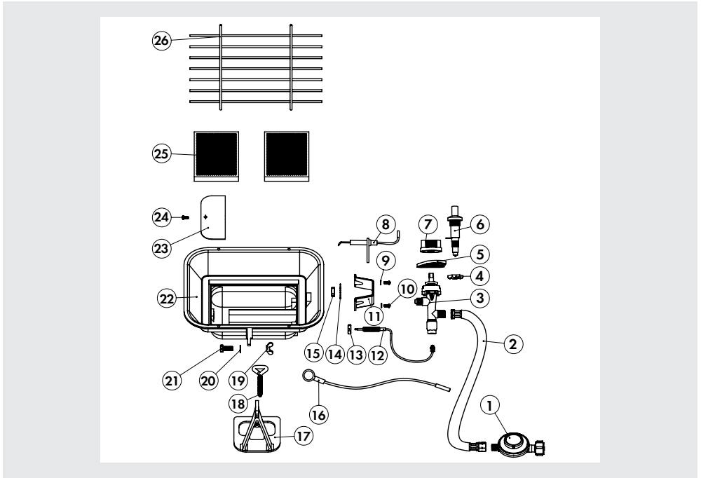
Abb. 4: Explosionszeichnung
