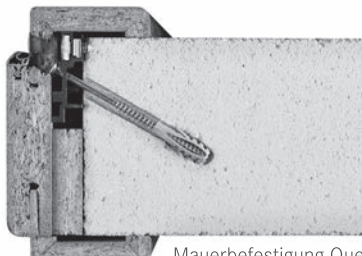
Mauerbefestigung Querschnitt
