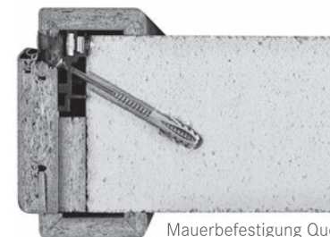
Mauerbefestigung Querschnitt
