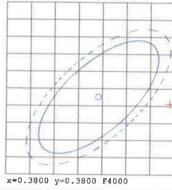
CIE1931色品图
