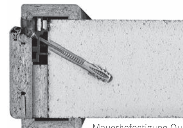
Mauerbefestigung Querschnitt
