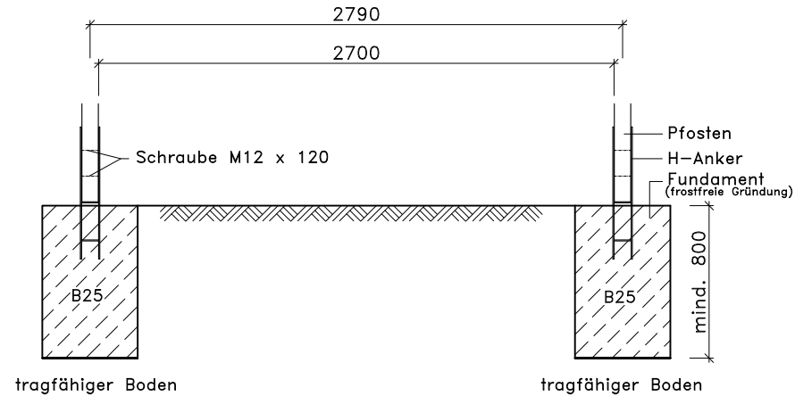
Schnitt B-B
